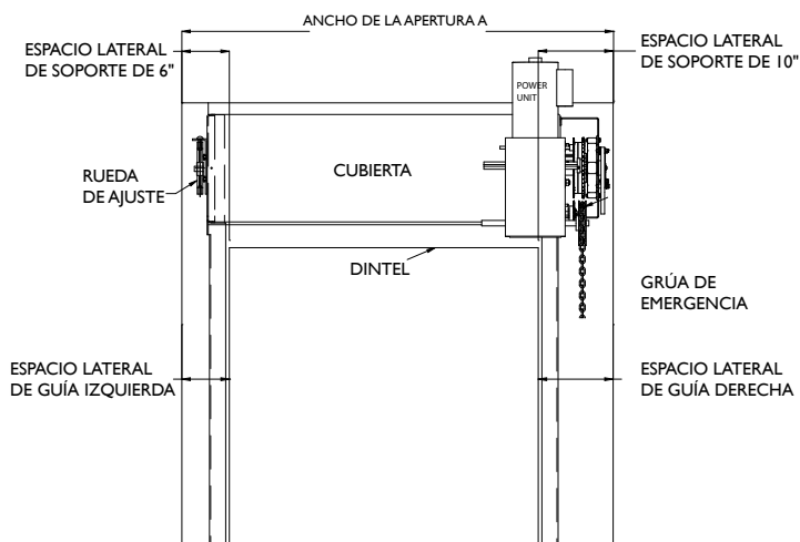
ELEVACIÓN DELANTERA
