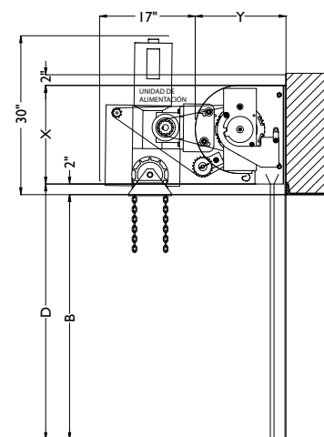
ELEVACIÓN LATERAL
