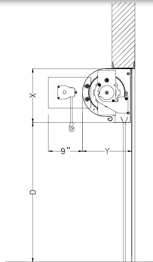
ELEVACIÓN LATERAL (DEBAJO DEL DINTEL)
