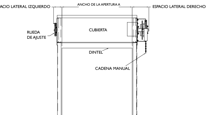
ELEVACIÓN DELANTERA
