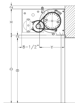
ELEVACIÓN LATERAL
