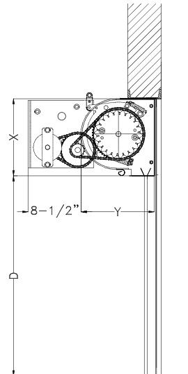
ELEVACIÓN LATERAL (DEBAJO DEL DINTEL)
