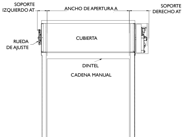
ELEVACIÓN DELANTERA
