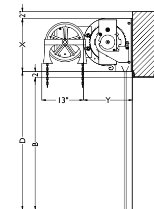
ELEVACIÓN LATERAL
