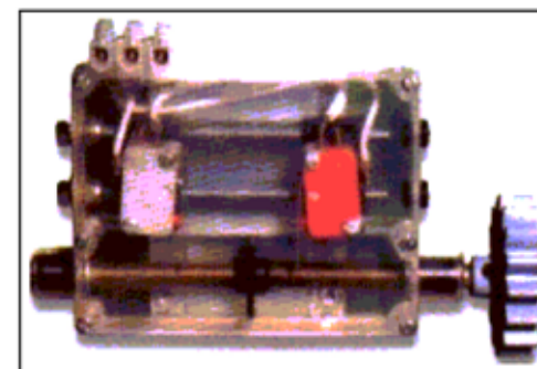
Caja de fines de carrera acoplado al motor
